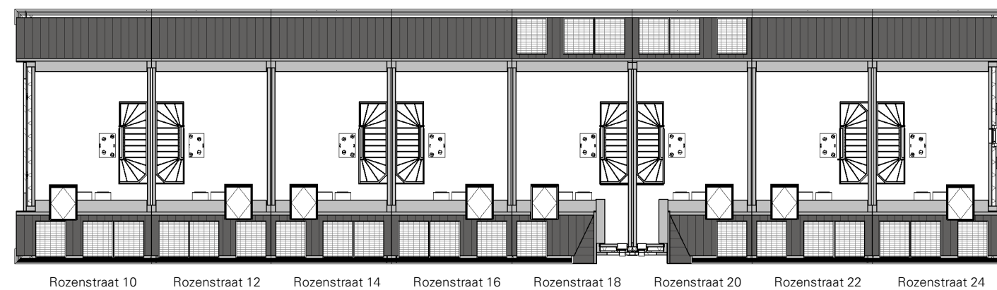
tweede verdieping
