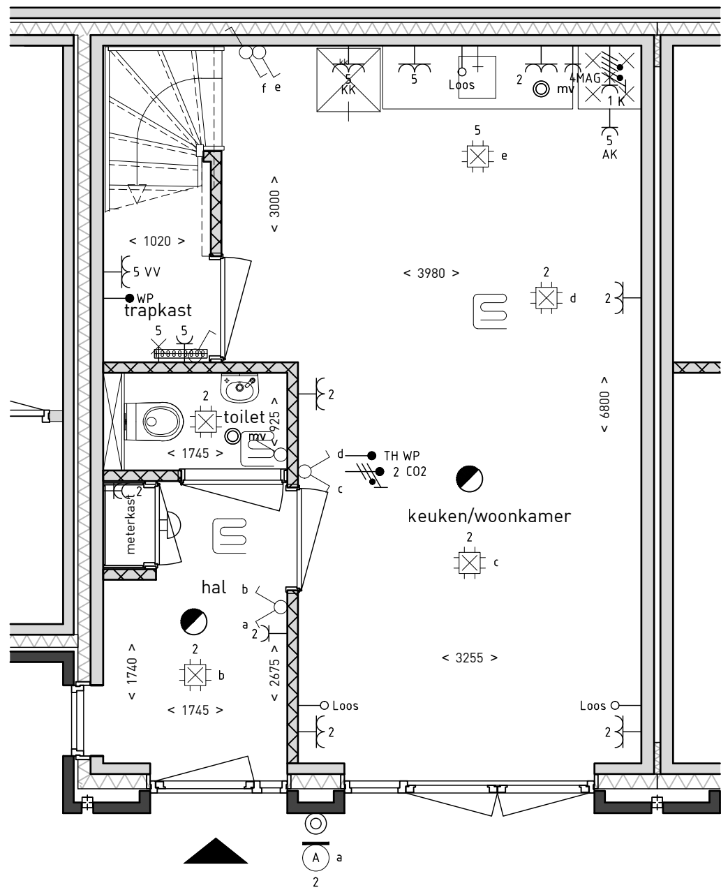
Molenstraat 46 begane grond 1:50
