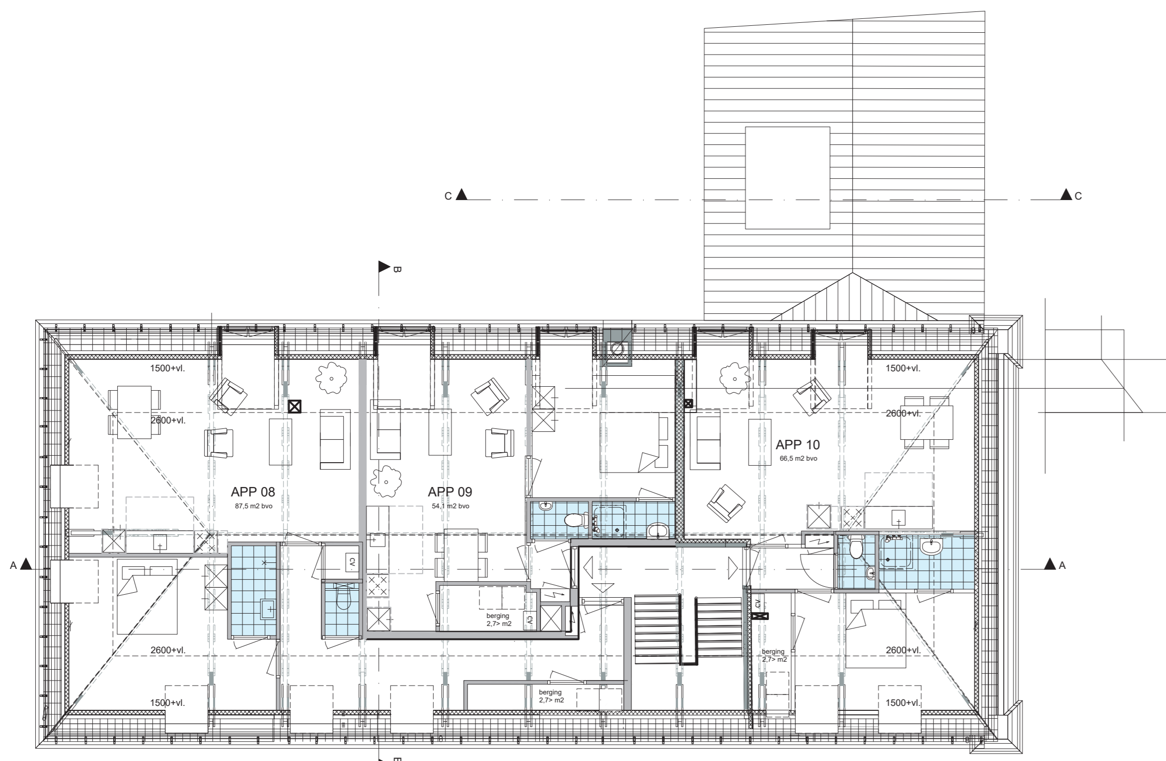
2e verdieping
