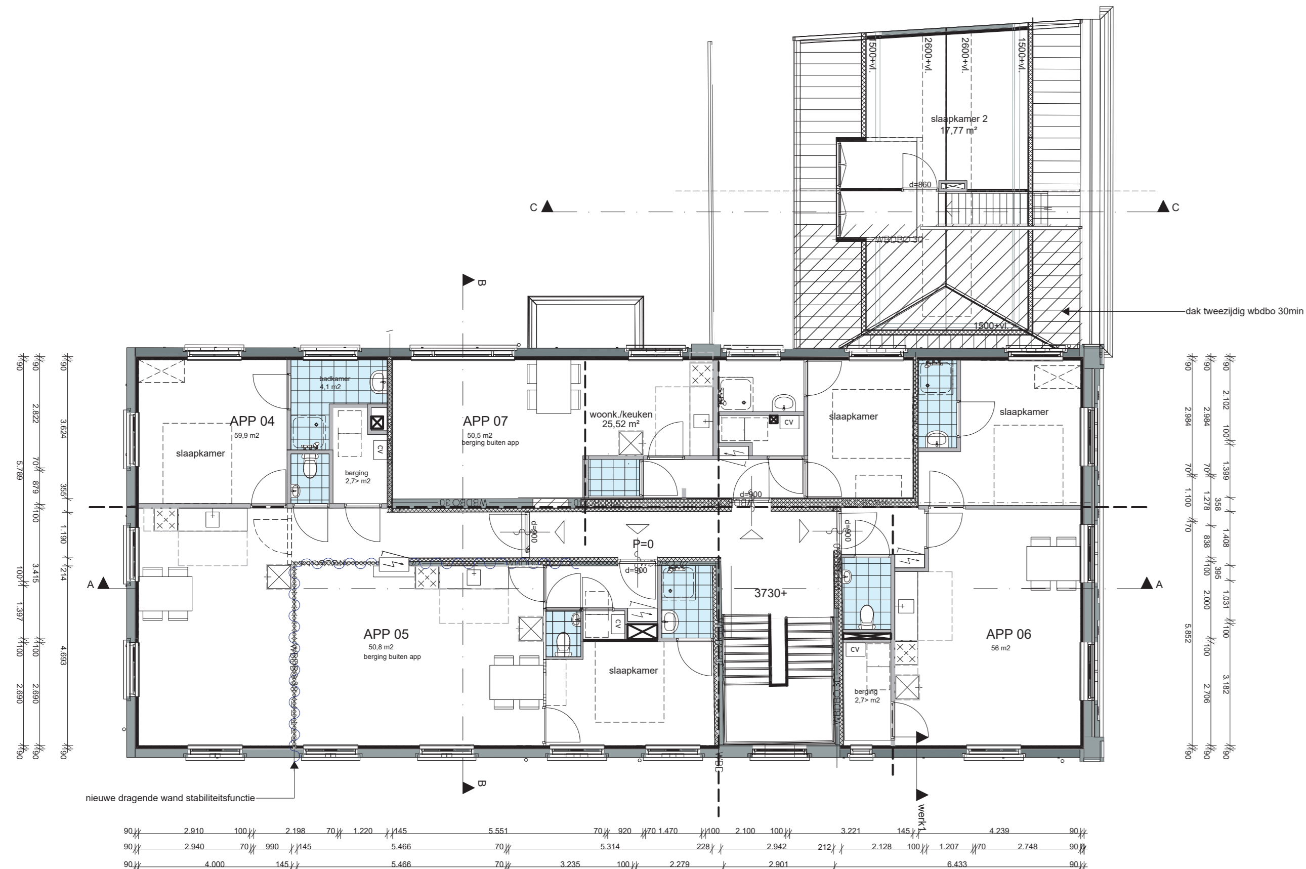
1e verdieping
