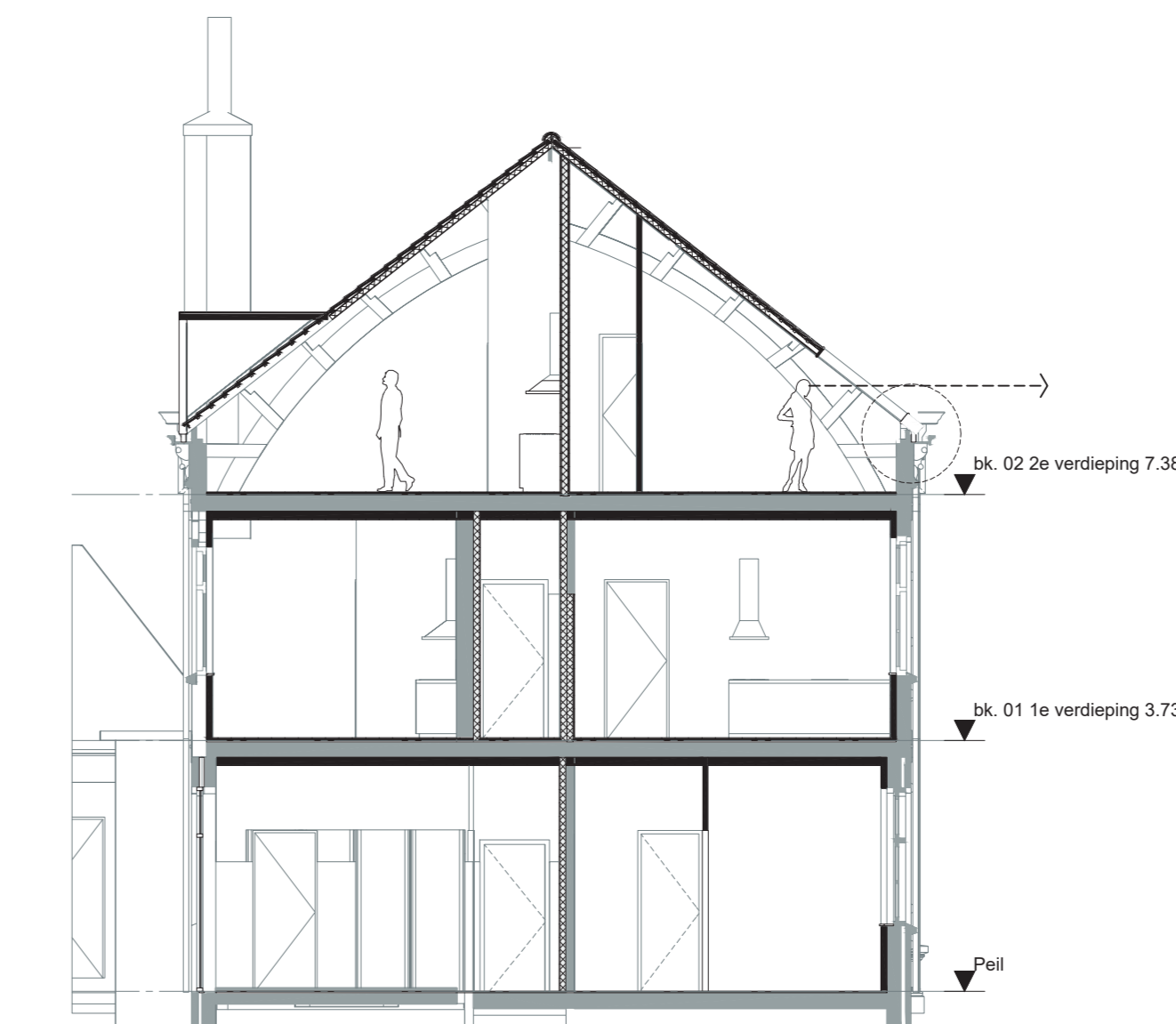
Doorsnede B-B
