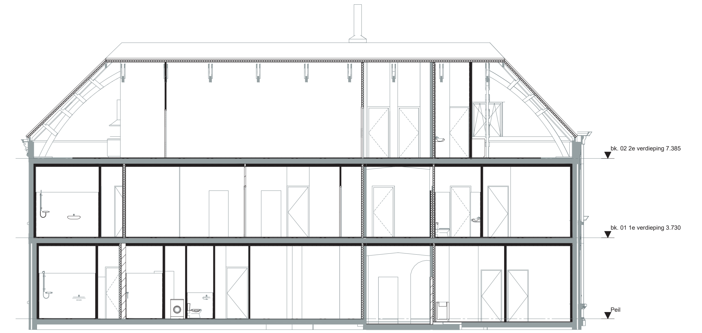
Doorsnede A-A
