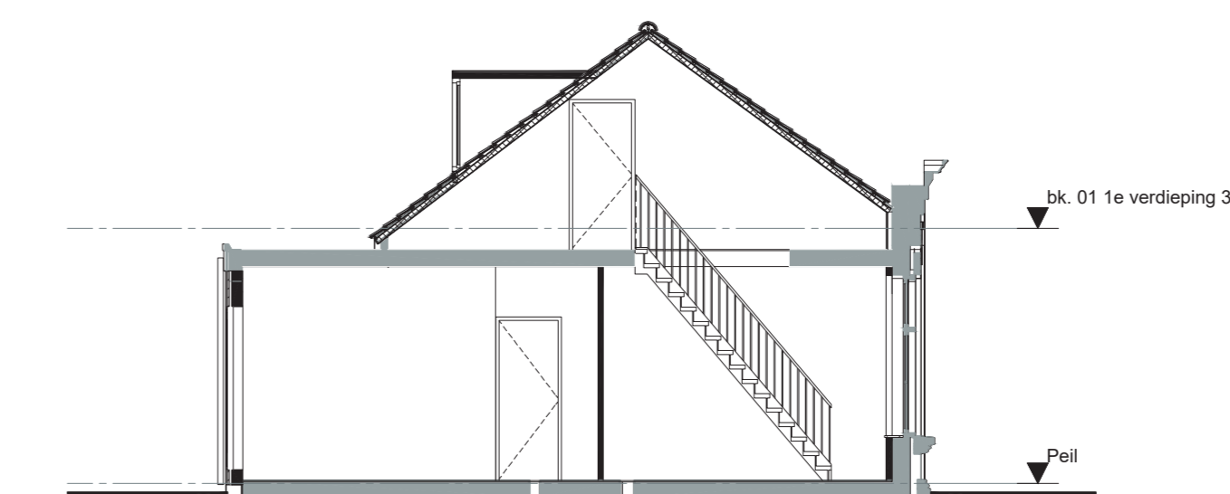
Doorsnede C-C
